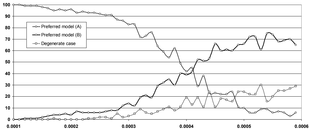
Pav. 4.2.3. Modelių (A) ir (B) efektyvumas, generavimas su modeliu (A), ant x ašies \nu/\alpha reikšmės, fiksuota reikšmė \nu/\alpha^2 = 32/(64000)^2 .
