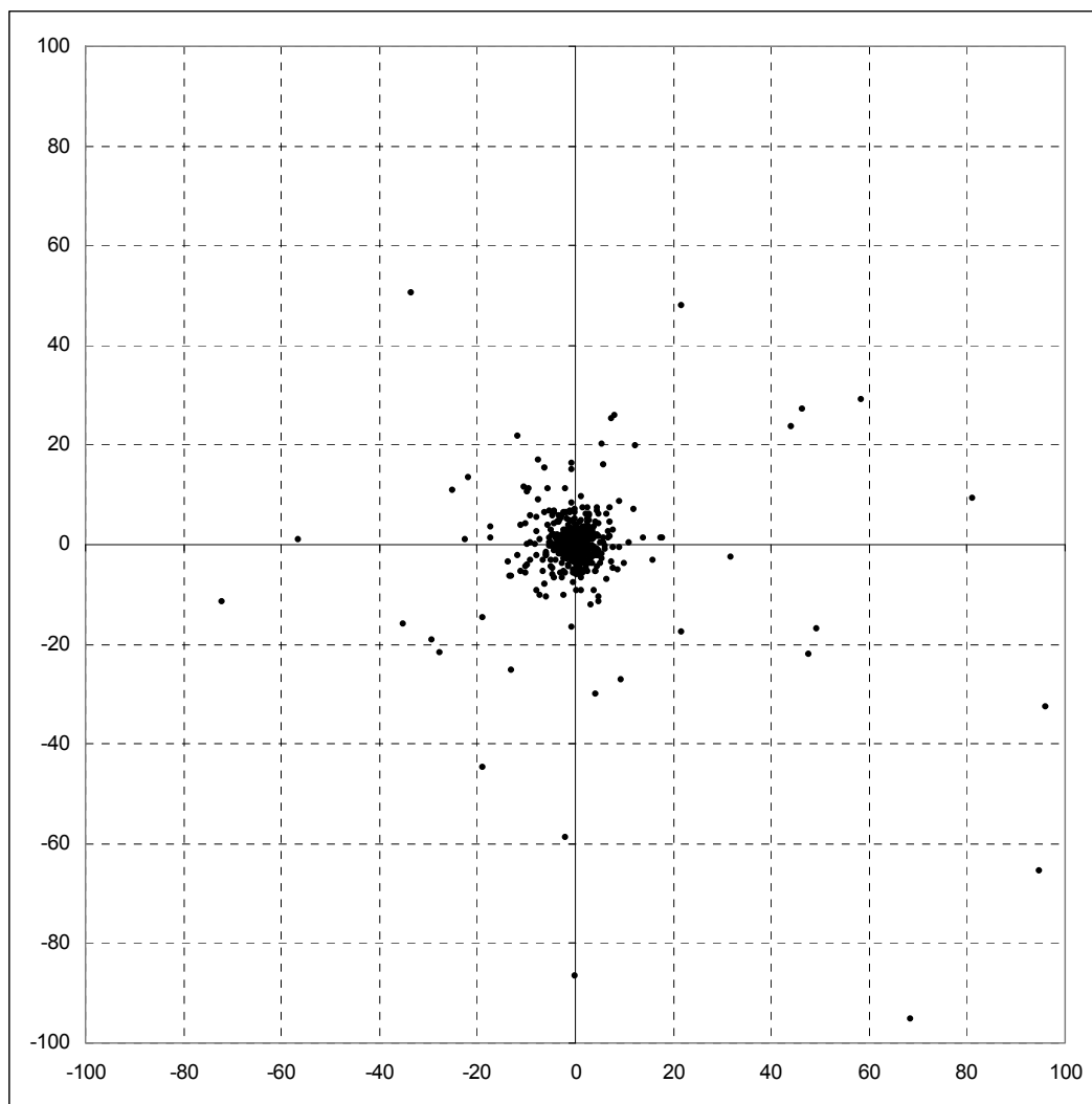
Pav. 3.2. Cauchy skirstinio pavyzdys, kai d = 2 (parodytos tik reikšmės, moduliu neviršijančios 100 kiekvienoje ašyje).
