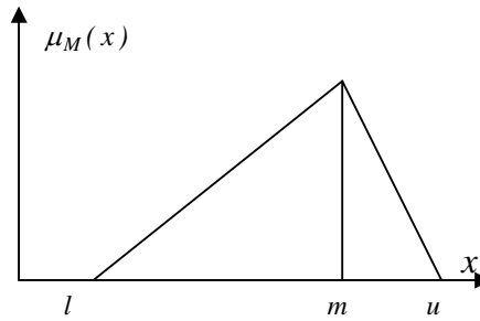
2.11 pav. Trikampių neraiškiųjų skaičių priklausymo funkcija
