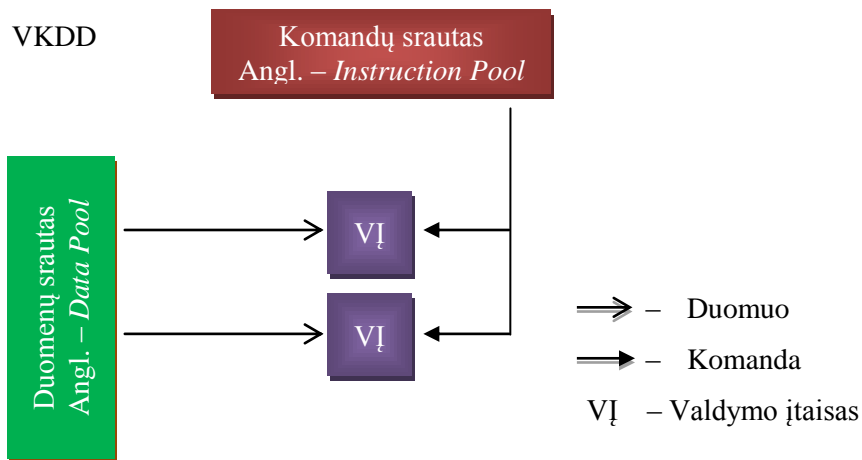
2.4 pav. Vienos Komandos Daug Duomenų srautų kompiuterio schema pagal Flyno taksonomiją
